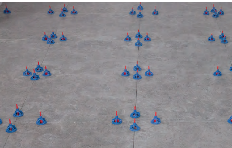
Aplicación Calzo Tornado / Tornado Clip application
